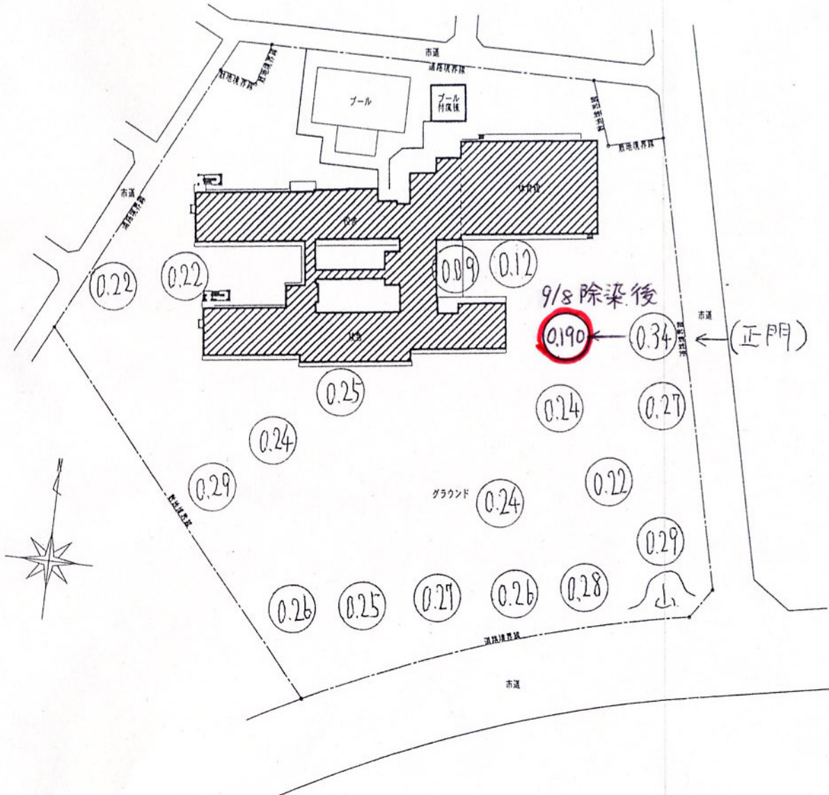
配置図 1:1,000
