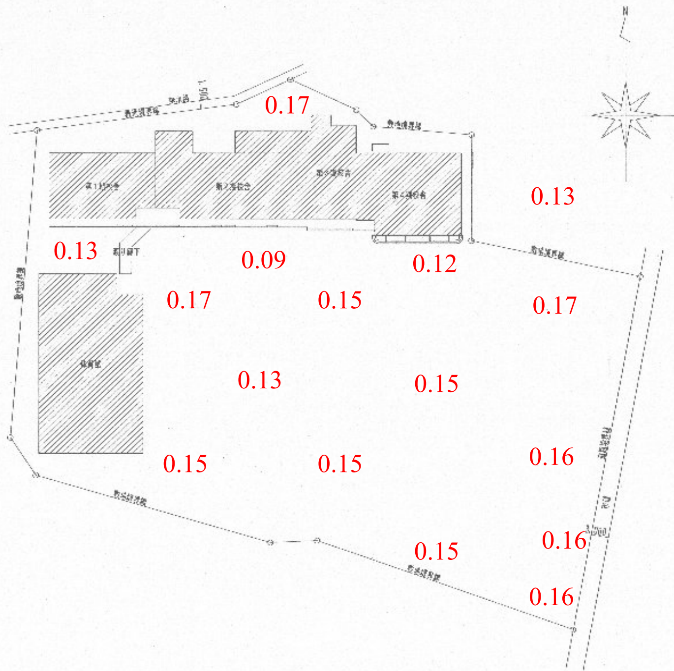
配置図 S=1/600
