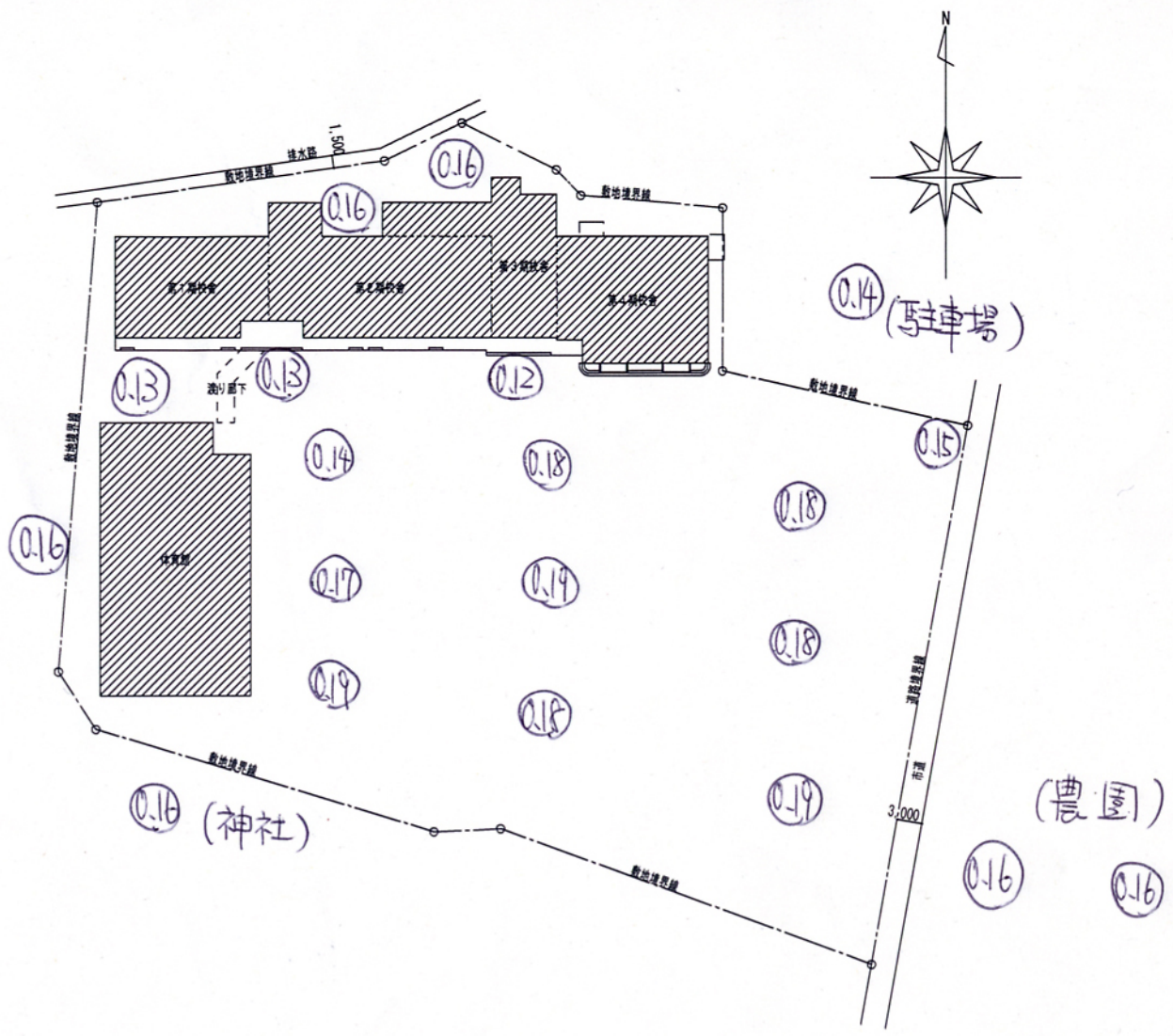
配置図 S=1/600
