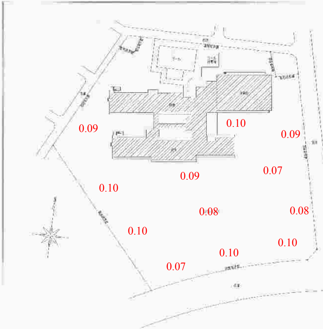
配置図 1
