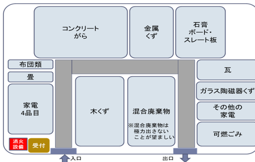
図表 3-12 一次仮置場の分別配置の例（再掲）
