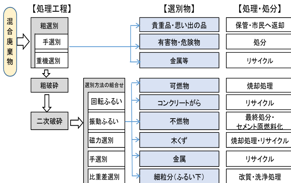
図表 3-14 混合廃棄物処理工程の例
