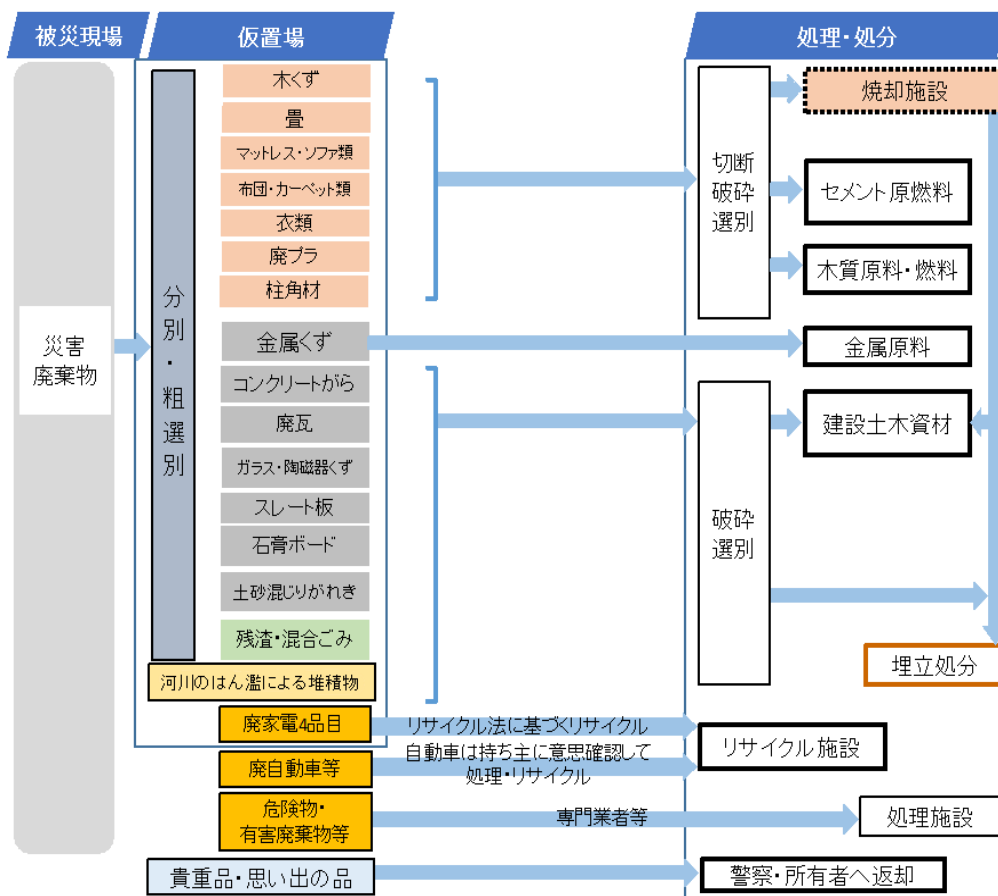
図表 3-7 災害廃棄物の種類別の処理方法（最大規模の場合）
