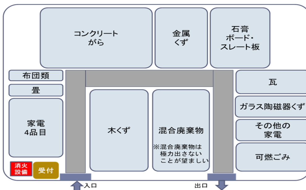
図表 3-9 一次仮置場の分別配置の例
