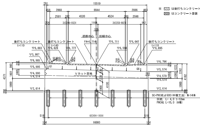
A 1 正面図
