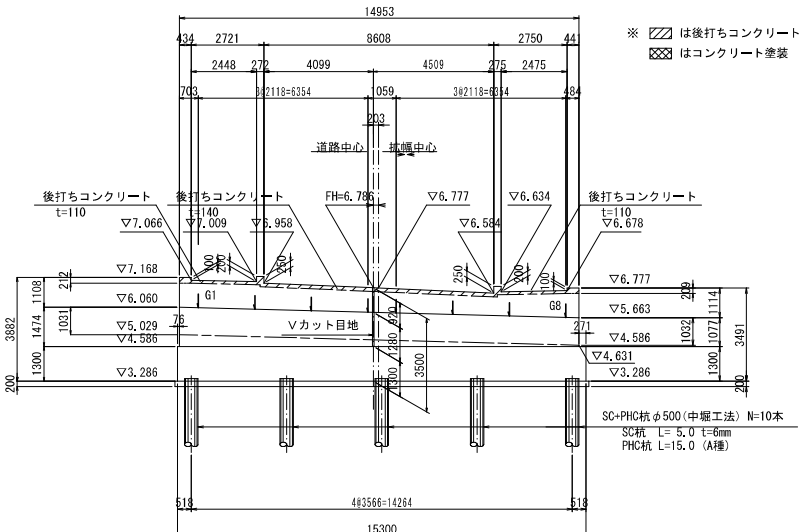
A 2 正面図
