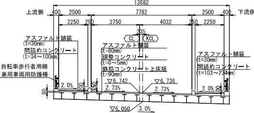
水路計画断面図
