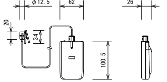
デジタルワイヤレスマイク(スティック型)
