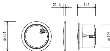
シーリングスピーカー
