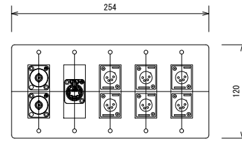
接続プレート
