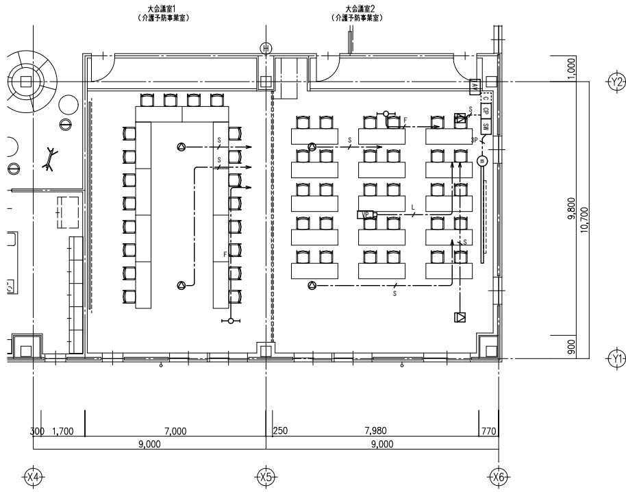
3階大会議室 AV設備 平面図 (A1:S=1/100)
