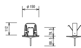
ワイヤレスマイク(天井埋込型)
