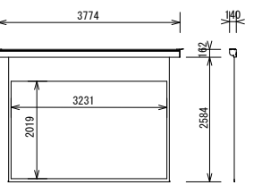
150型電動巻上スクリーン
