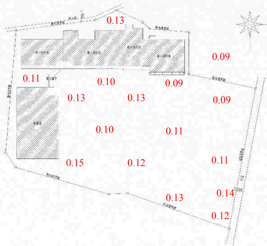
配置図 5=1/600
