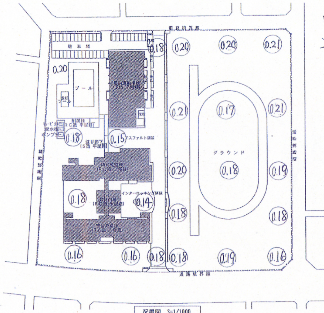
配置図 S=1/1000
