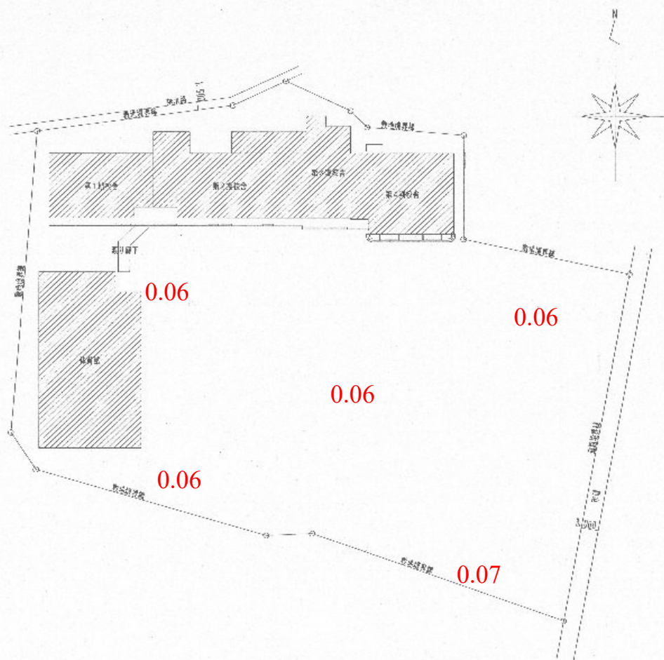
配置図 S=1/600
