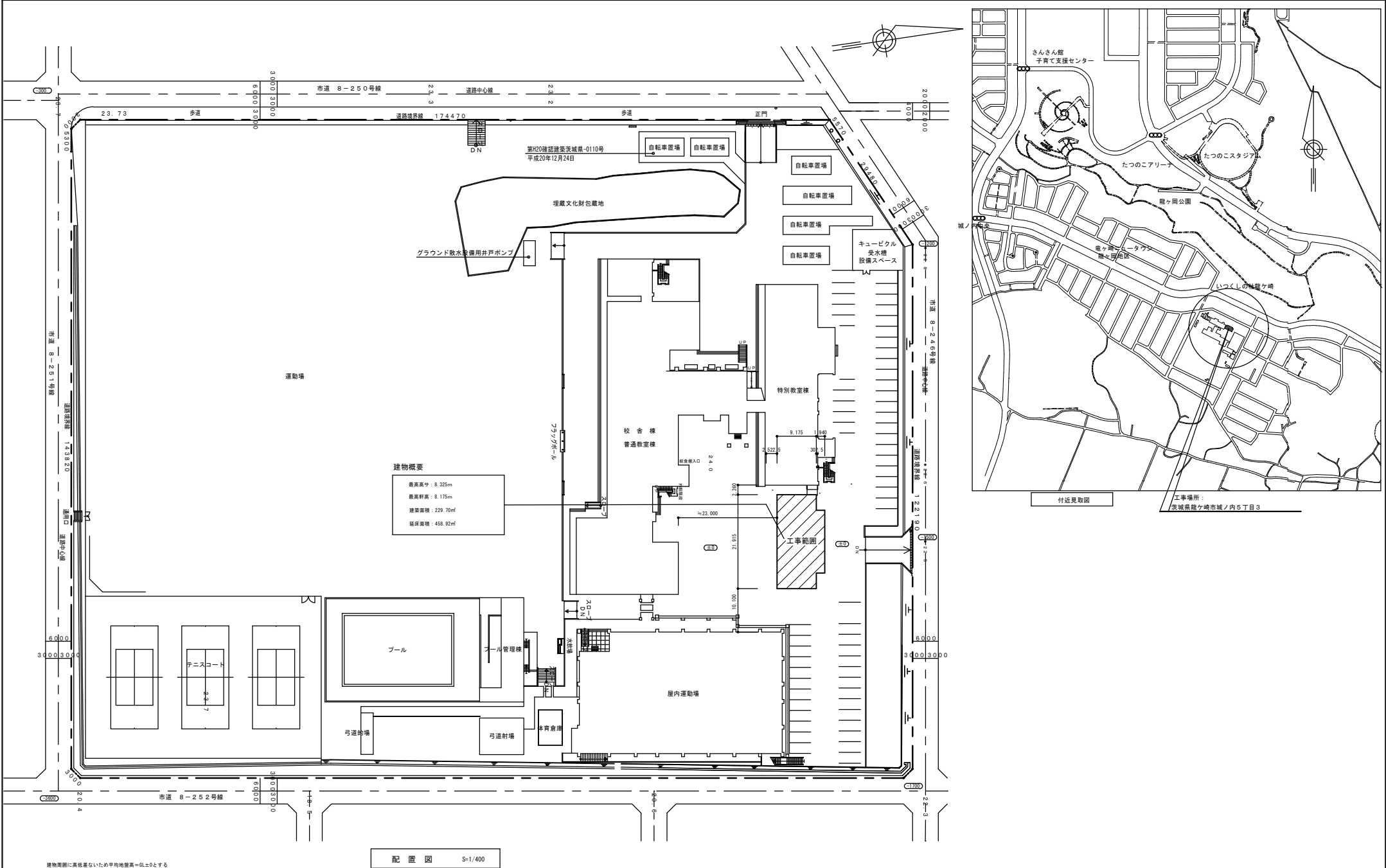
配置図 S=1/400
