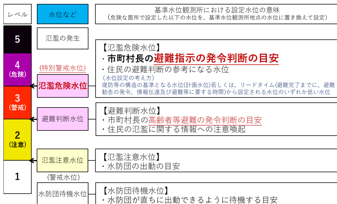
基準水観測所における設定水位の意味（表1）
